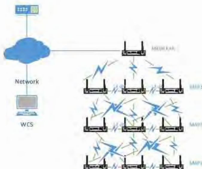
Slika 2.9 Ravna WMN mreža
