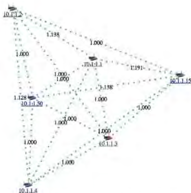
Slika 2.2 Potpuno konektovana mesh mreža
