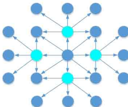
Slika 5.3 OLSR: Smanjen protok sa MPR selekcijom
