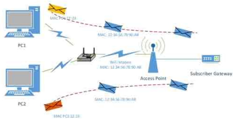
Slika 2.11 Dodeljivanje potkanala MAC protokola
