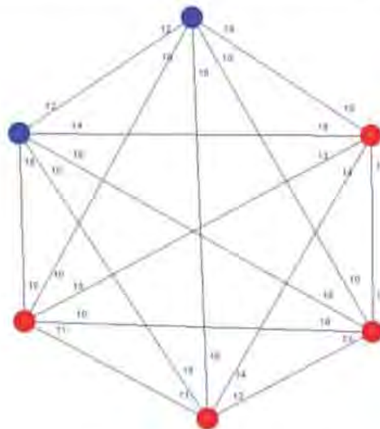
Slika 7.9 Klasterizacija čvorova
