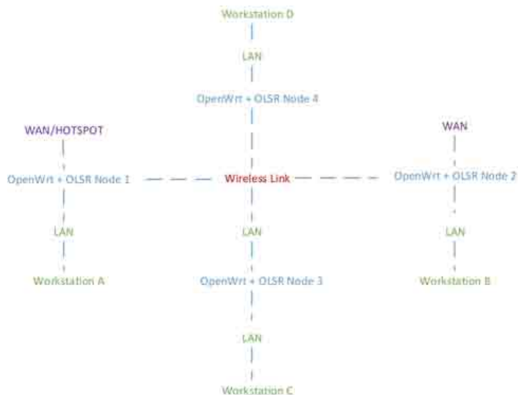
Slika 5.4 Konfiguracija WMN mreže sa četiri čvora
