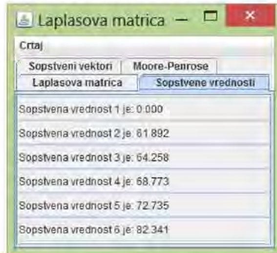
Slika 7.4 Sopstvene vrednosti Laplasove matrice
