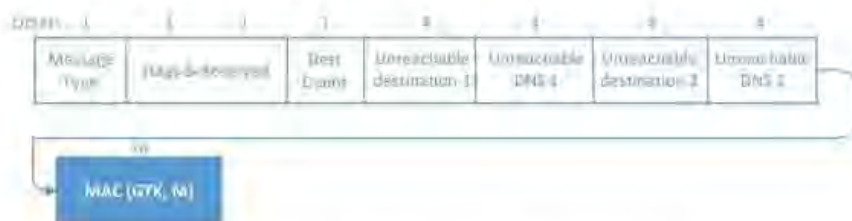
Slika 4.10 Struktura RERR poruke u SEAODV protokolu
