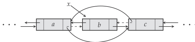
Slika 4.10: Uklanjanje čvora x iz dvostruko povezane liste.
