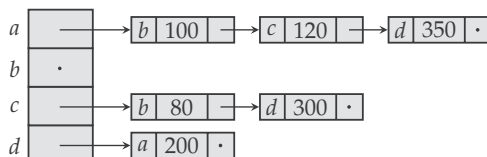
Slika 8.3: Niz listi susedstva za težinski graf na slici 8.1.
