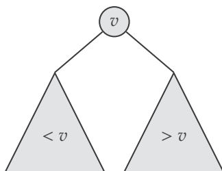
Slika 6.9: BSP svojstvo svakog čvora binarnog stabla pretrage.
