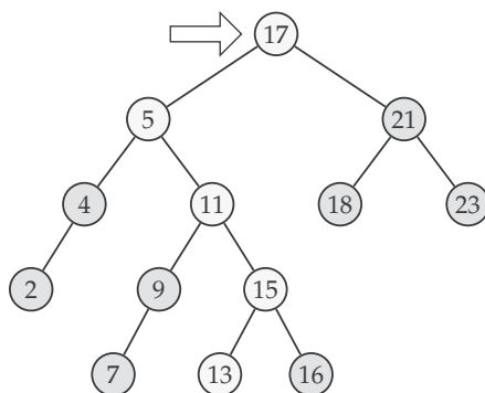
Slika 6.11: Traženje čvora 13 u datom binarnom stablu pretrage.
