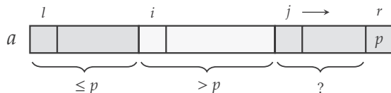
Slika 5.7: Pivotiranje sa poslednjim elementom podniza.
