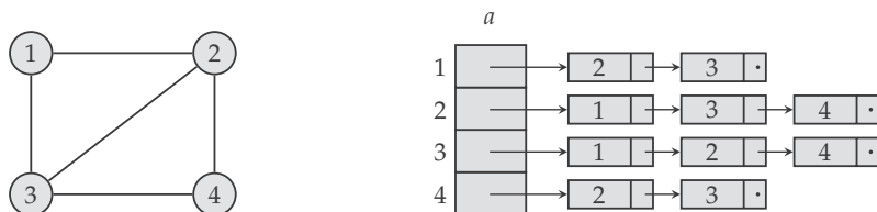
Slika 7.10: Neusmeren graf predstavljen listama susedstva.
