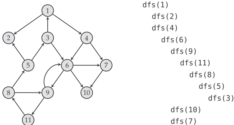
Slika 7.16: Izvršavanje algoritma dfs od čvora 1 datog usmerenog grafa.
