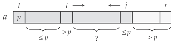
Slika 5.6: Pivotiranje sa prvim elementom podniza.
