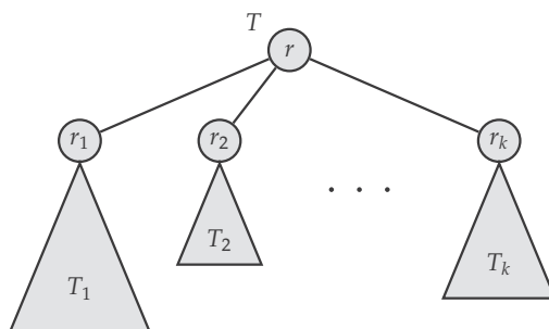
Slika 6.2: Rekurzivna definicija stabla T .
