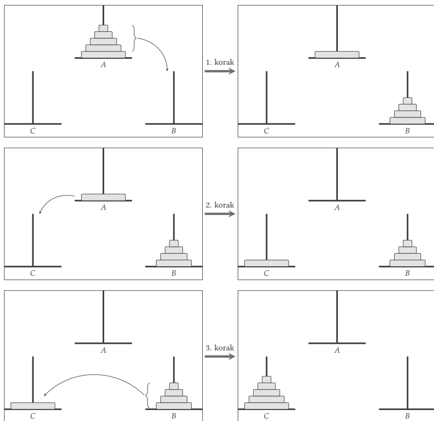
Slika 5.3: Rekurzivno rešenje igre Hanojskih kula.
