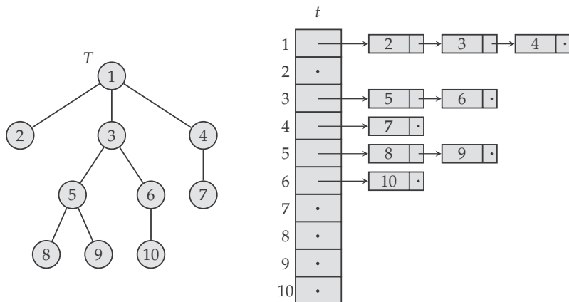
Slika 6.4: Predstavljanje stabla listama dece čvorova.
