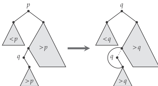
Slika 6.16: Opšti slučaj uklanjanja unutrašnjeg čvora p sa dvoje dece iz binarnog stabla pretrage.
