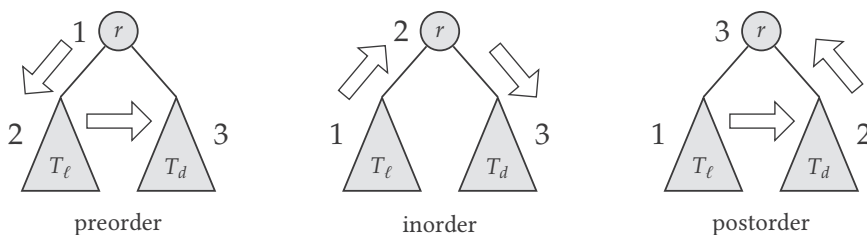
Slika 6.7: Tri načina obilaska binarnog stabla.
