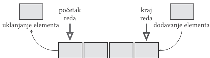
Slika 4.15: Osnovne operacije sa elementima reda za čekanje.
