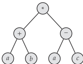
Slika 6.3: Stablo izraza (a + b) * (a - c) .
