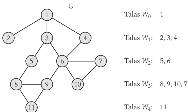
Slika 7.11: Talasi pretrage u širinu datog grafa G od početnog čvora 1.
