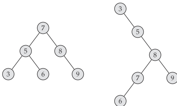
Slika 6.10: Dva binarna stabla pretrage sa istim ključevima.
