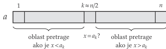
Slika 3.3: Binarna pretraga.
