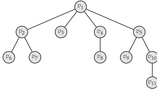
Slika 6.1: Korensko stablo.
