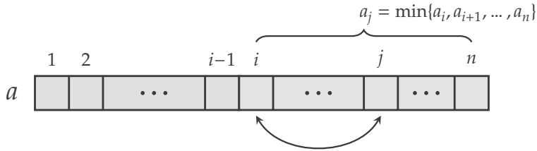
Slika 2.4: Sortiranje izborom.
