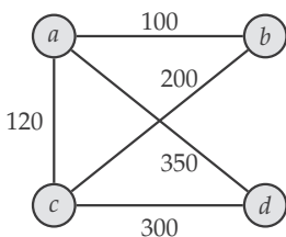
Slika 8.1: Težinski graf.
