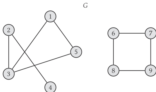
Slika 7.4: Nepovezan graf.
