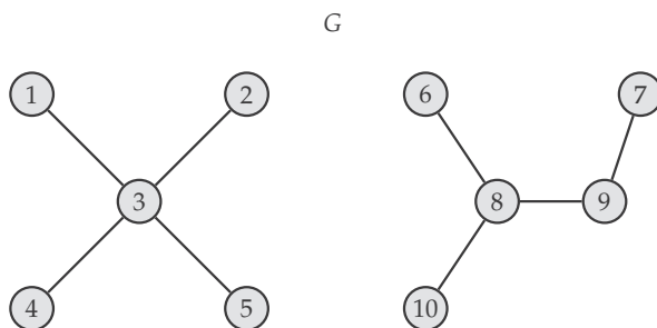
Slika 7.6: Šuma.
