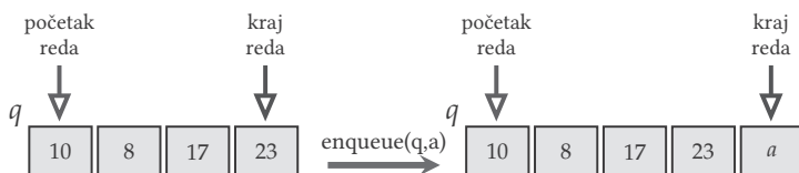
Slika 4.16: Operacija dodavanja elementa redu za čekanje.
