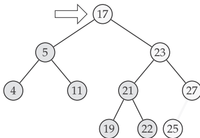
Slika 6.12: Dodavanje čvora 25 datom binarnom stablu pretrage.
