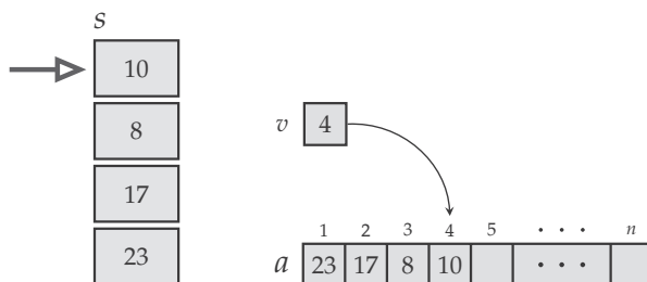
Slika 4.14: Stek s predstavljen nizom a .
