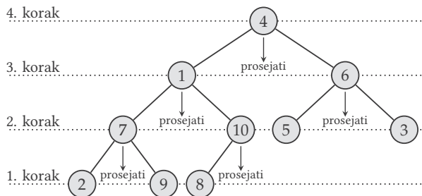
Slika 6.25: Konstruisanja hipa od stabla sa neuređenim čvorovima.
