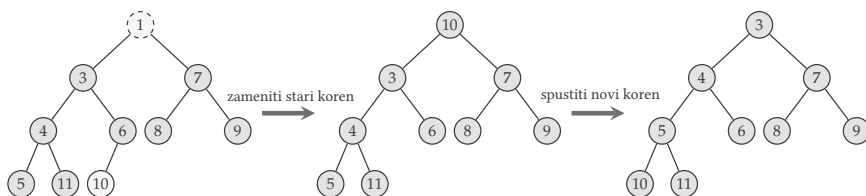
Slika 6.22: Uklanjanje najmanjeg čvora iz hipa.
