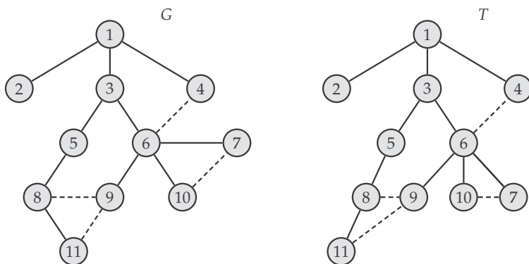
Slika 7.12: Stablo T dobijeno pretragom u širinu datog grafa G od čvora 1.
