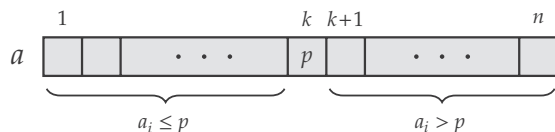
Slika 5.5: Podela niza kod sortiranja razdvajanjem.
