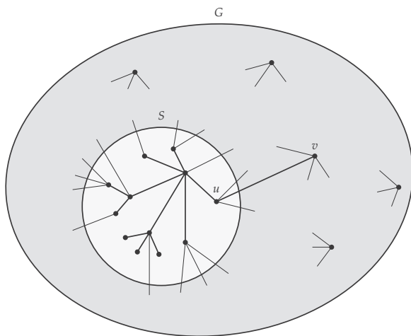
Slika 8.7: Jedna iteracija Primovog algoritma.
