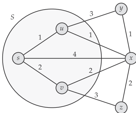
Slika 8.10: Primer izvršavanja Dijkstrinog algoritma.
