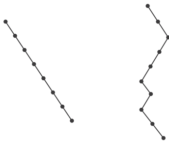
Slika 6.19: Najgora binarna stabla pretrage.
