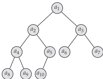
Slika 6.24: Predstavljanje hipa sa 10 čvorova pomoću niza.
