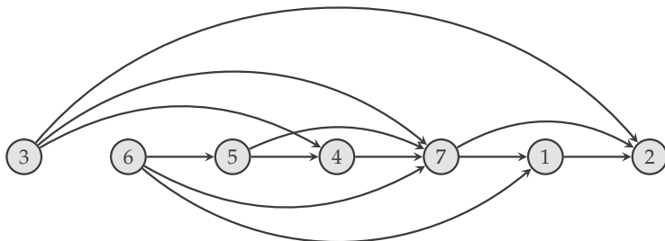
Slika 7.21: Topološki redosled grafa na slici 7.18.
