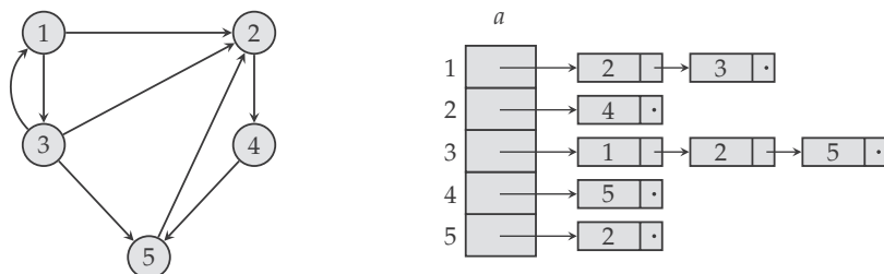
Slika 7.9: Usmeren graf predstavljen listama susedstva.
