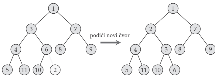
Slika 6.23: Dodavanje novog čvora u hip.
