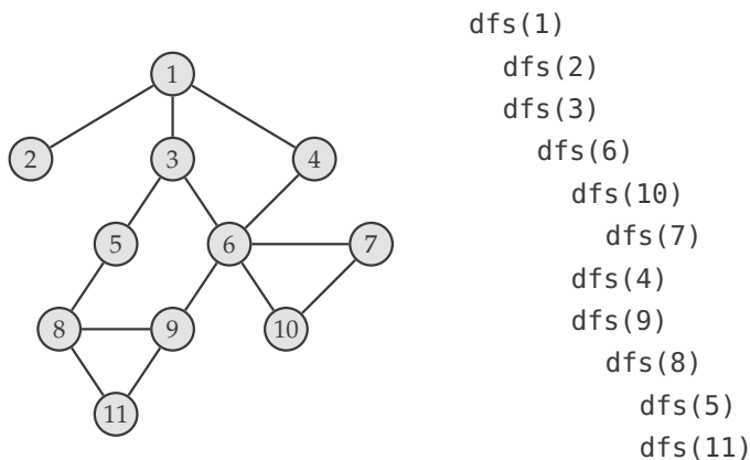
Slika 7.13: Izvršavanje algoritma dfs od čvora 1 datog grafa.
