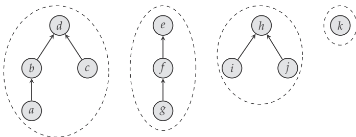
Slika 6.27: Disjunktne skupove predstavljene kolekcijom stabala.
