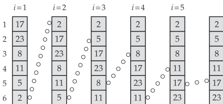
Slika 2.2: Sortiranje zamenjivanjem.
