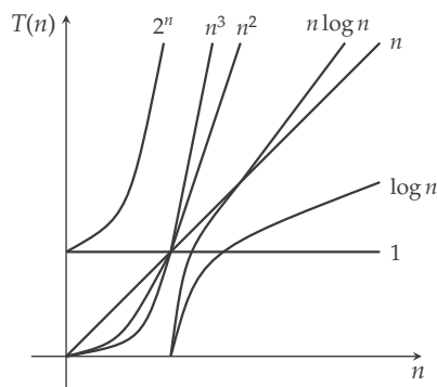
Slika 3.4: Tipične funkcije za vremena izvršavanja algoritama.
