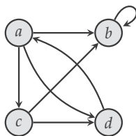
Slika 7.2: Usmeren graf.
