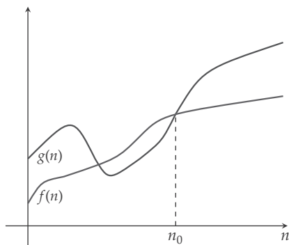
Slika 3.5: f(n) = O(g(n)) .
