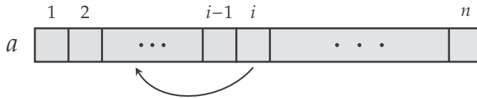
Slika 2.3: Sortiranje umetanjem.
