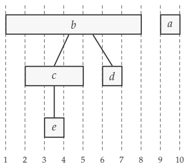
Slika 7.22: Intervali trajanja poziva algoritma dfs prikazani na vremenskoj osi tokom višestruke pretrage u dubinu grafa na slici 7.19.
