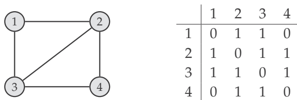
Slika 7.8: Neusmeren graf i njegova matrica susedstva.
