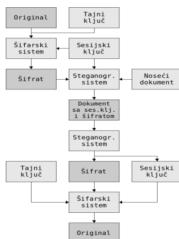
Slika 2. – Put podataka koji se štite kroz sistem
